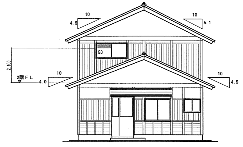
東面立面図 S=1/100
