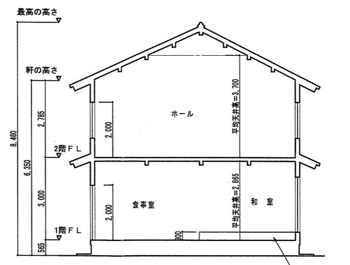
b~b' 断面図 S=1/100
