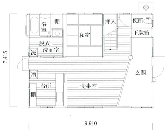
1階平面図
